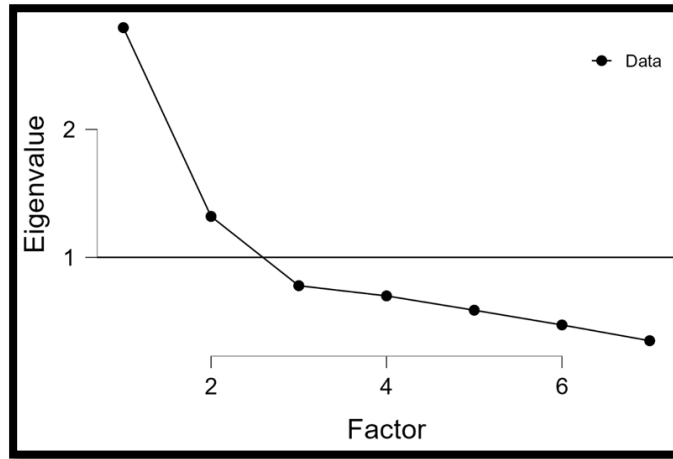
Şekil 1. Yamaç Eğim (Scree Plot) Grafiği
