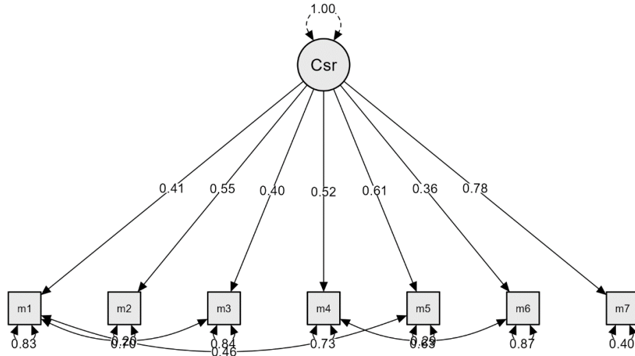
Şekil 2. Faktör Yükleri
