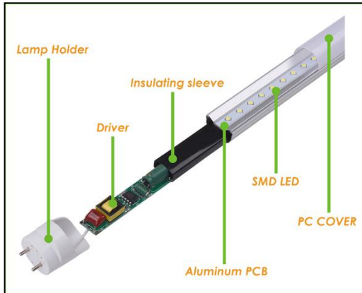
Şekil.2 LED Floresan Lambanın yapısı [5]
