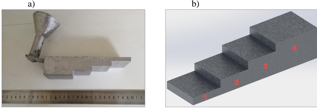
Şekil 3. a) Döküm numunelere ait örnek görüntü ve b) Döküm numunesinin incelenmek üzere bölge kodlarının gösterimi
