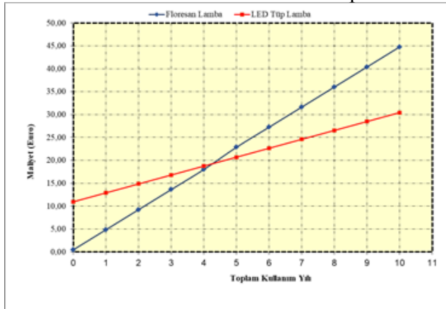
Grafik.3 Günlük 8 saat kullanımda Toplam Kullanım Yılı-Toplam Maliyet deęiřimi.
