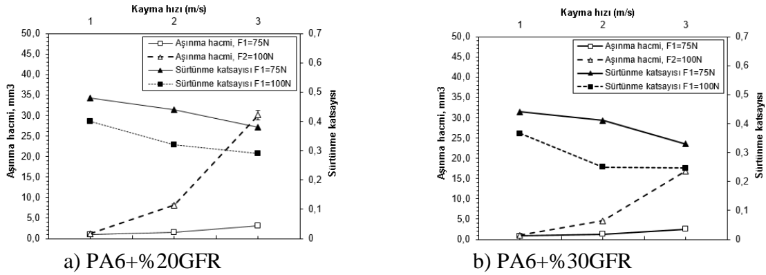
Şekil 2. Cam elyaf miktarına bağlı olarak aşınma ve sürtünme özelliklerindeki değişim
