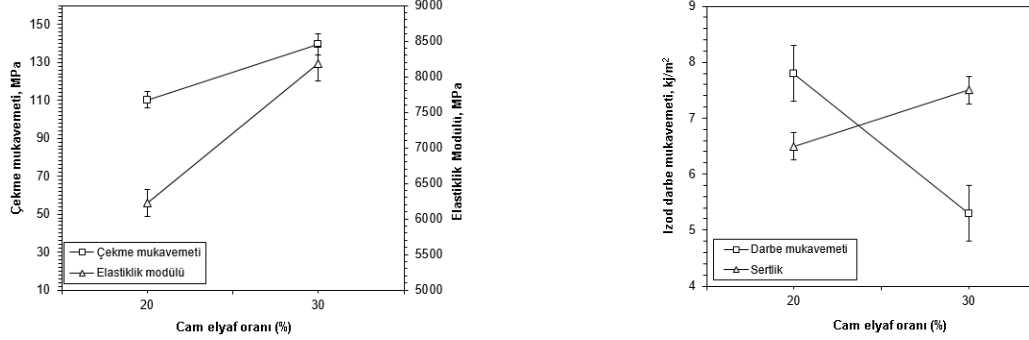
a) Çekme dayanımı-Elastiklik modülü değişimi b) Darbe dayanımı-sertlik değişimi
