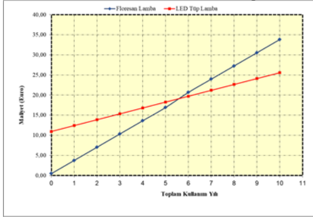
Grafik.2 Günlük 6 saat kullanımda Toplam Kullanım Yılı-Toplam Maliyet deęiřimi.
