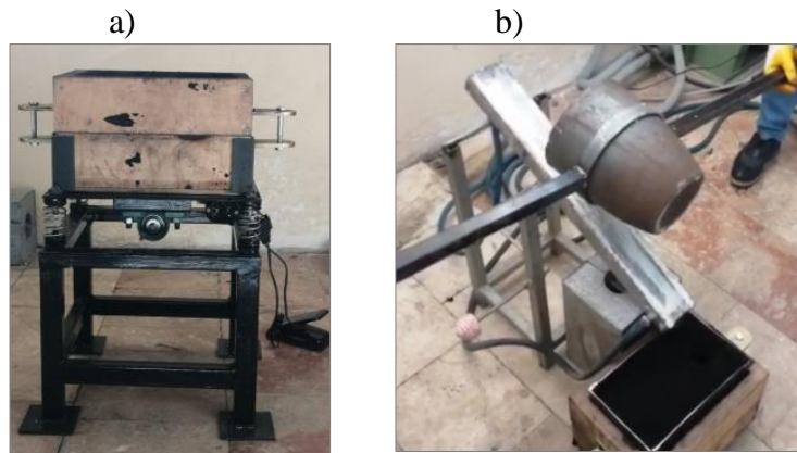
Şekil 2. a) mekanik titreşim altında katılaşma için kullanılan deney düzeneği, b) eğimli soğutma plakası deney düzeneği
